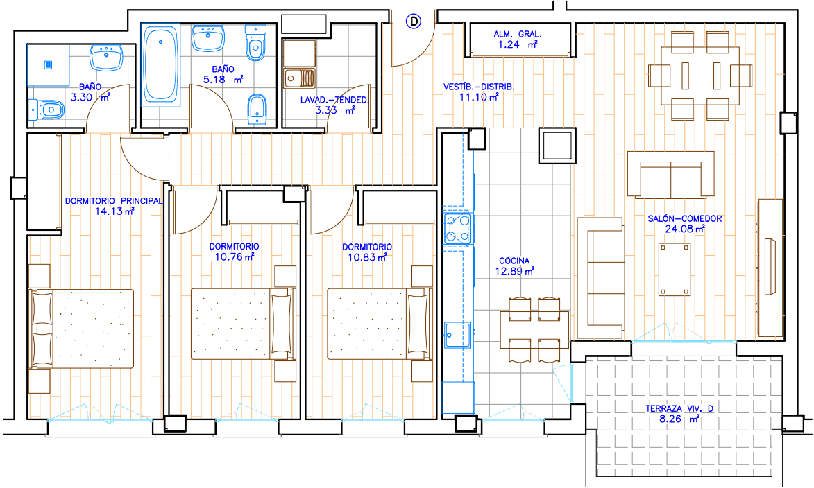
DISTRIBUCIÓN ALTERNATIVA CON SALÓN Y COCINA UNIDOS esc 1/100
